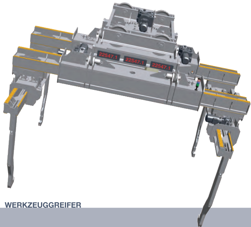
3-D Konstruktionsdarstellung eines Werkzeuggreifers mit Wegmeßsystem und Digitalanzeigen. (Abb. oben)
